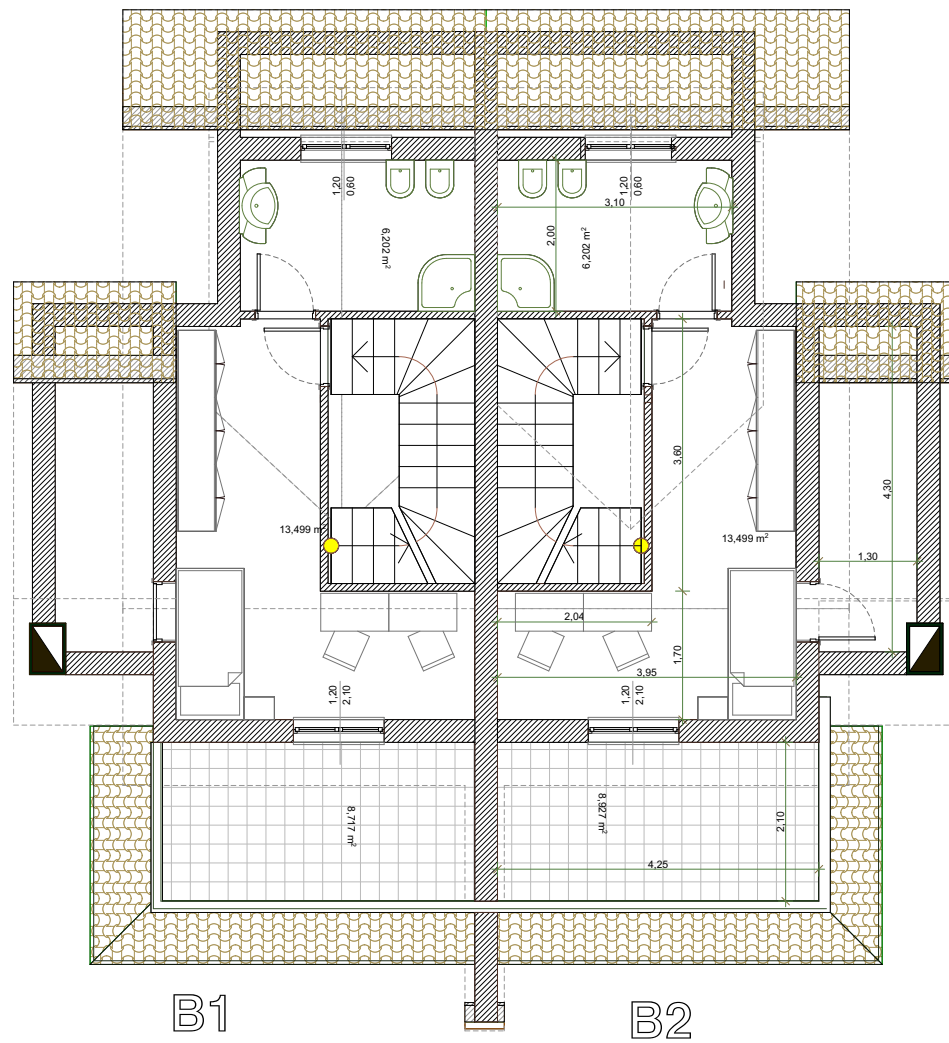
PIANO SECONDO SCALA 1:100
